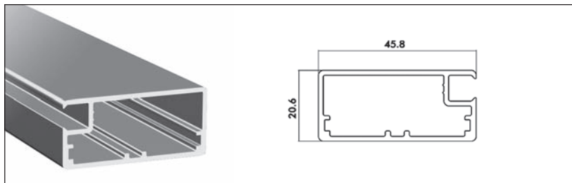
■ SAS 006 keretprofil
