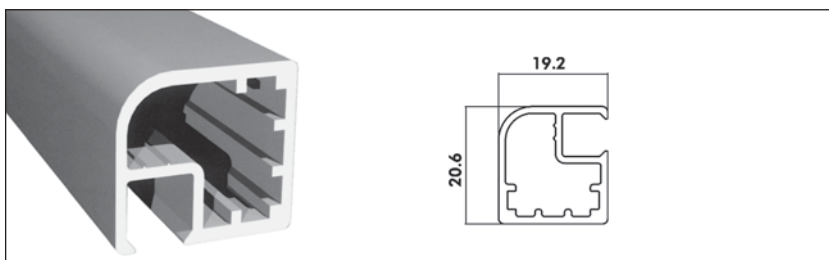
■ SAS 005 keretprofil
